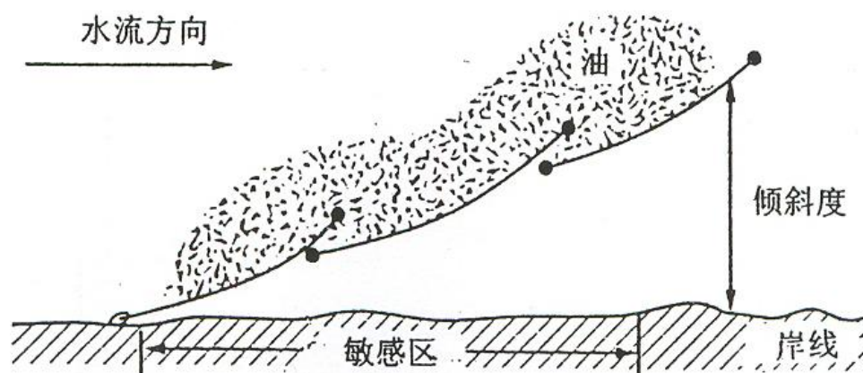
图 4-4 转移围栏
