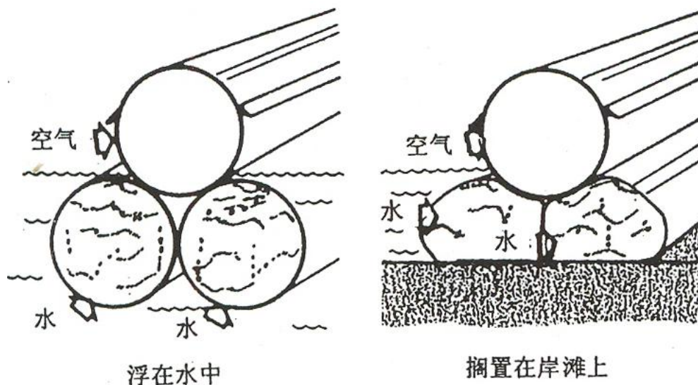
图 4-5 拦截围栏
