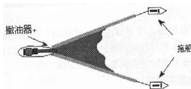
图 5-9 三船开口 U 形布放围油栏
