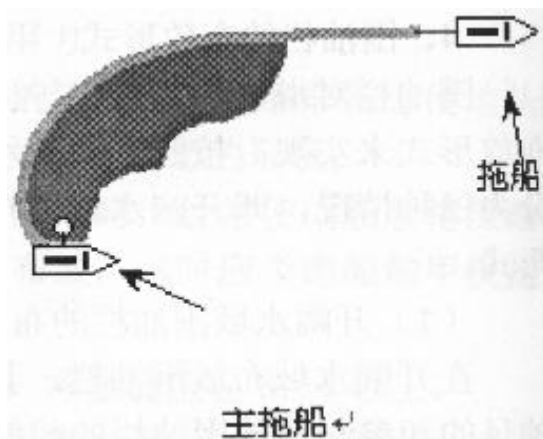
图 5-7 两船 J 形布放围油栏
